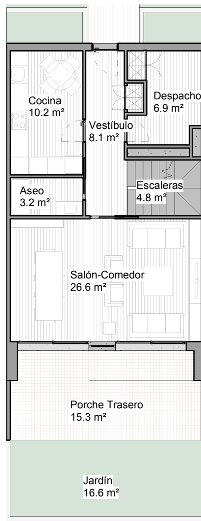
PLANTA BAJA 1 : 125
