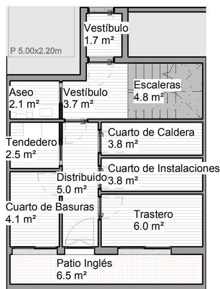
PLANTA SÓTANO 1 : 125
