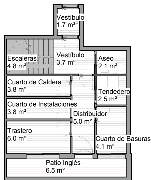
PLANTA SÓTANO 1 : 125
