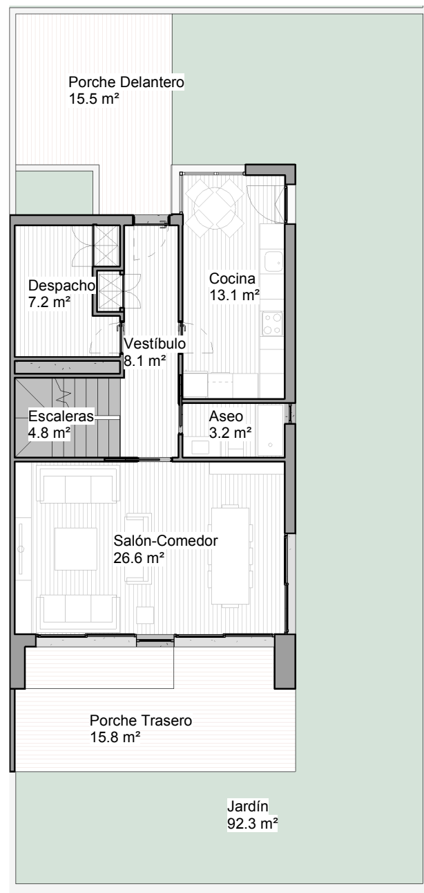
PLANTA BAJA 1 : 125
