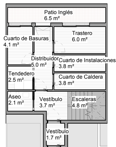
PLANTA SÓTANO
