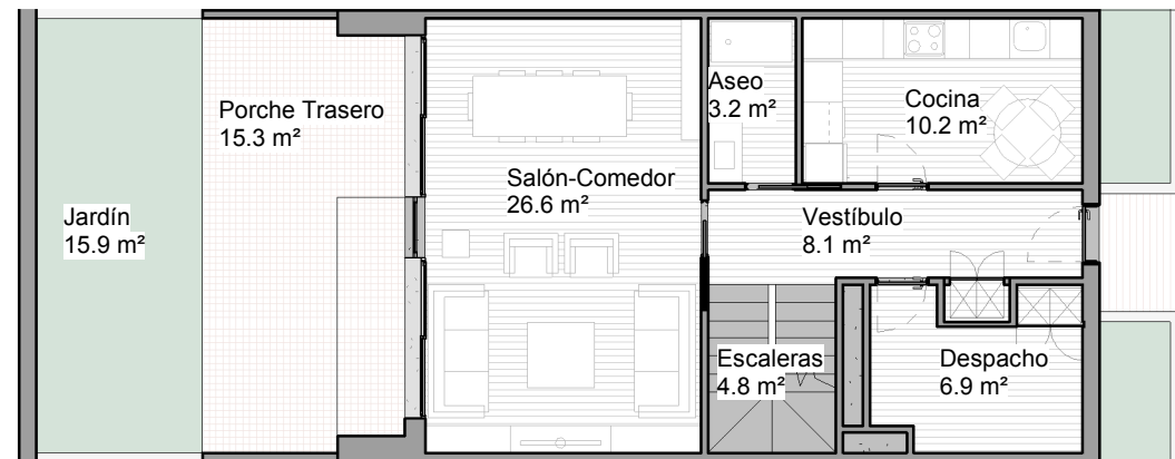
PLANTA BAJA 1 : 125
