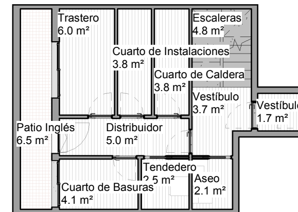
PLANTA SÓTANO 1 : 125
