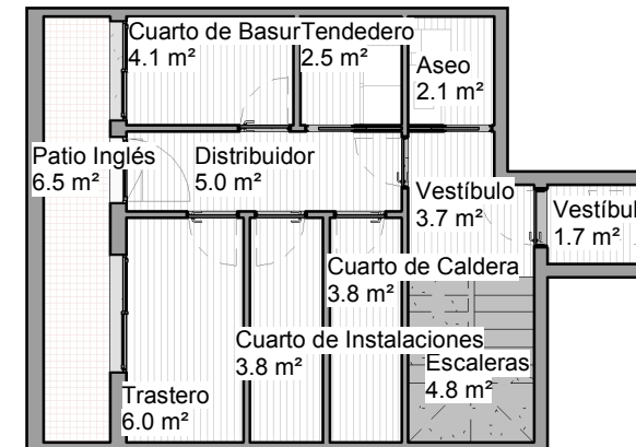
PLANTA SÓTANO 1 : 125
