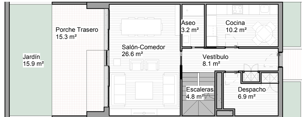
PLANTA BAJA 1 : 125
