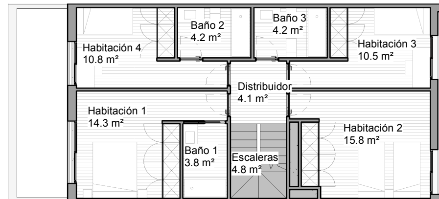
PLANTA PRIMERA 1 : 125
