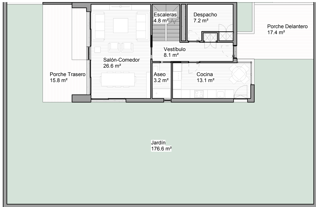
PLANTA BAJA 1 : 125
