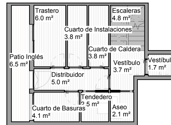
PLANTA SÓTANO 1 : 125
