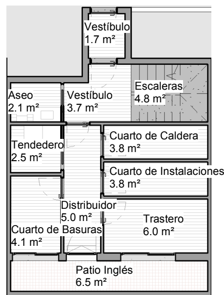
PLANTA SÓTANO
