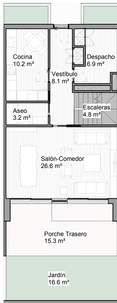
PLANTA BAJA
